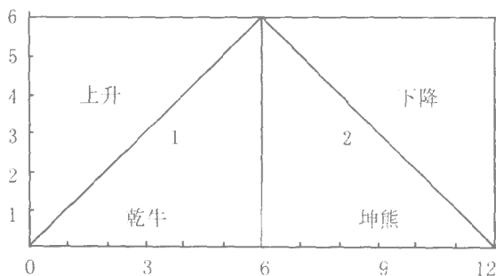
图 7-1 股市及经济发展初期的牛熊二波性
